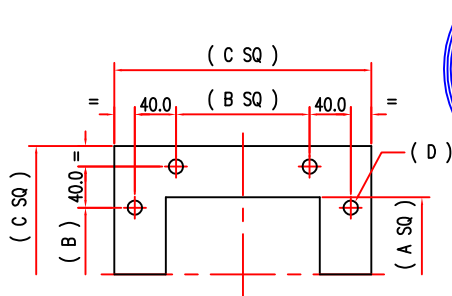
AL 152 SQ TOP & BOTTOM FLANGE
