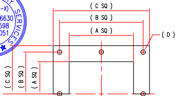
AL 200 SQ TOP & BOTTOM FLANGE
